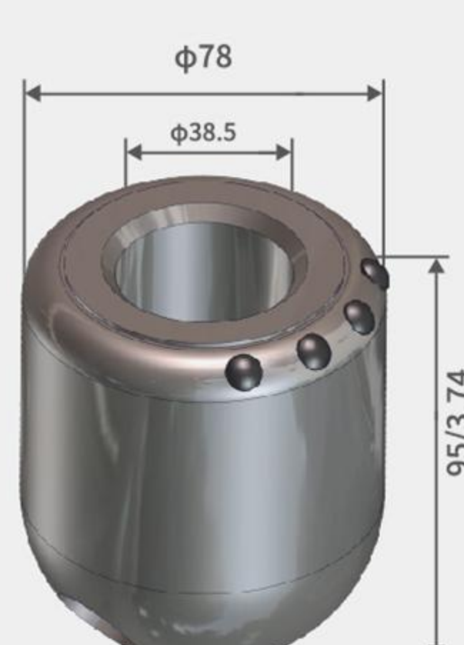
合金大圆座78-95
