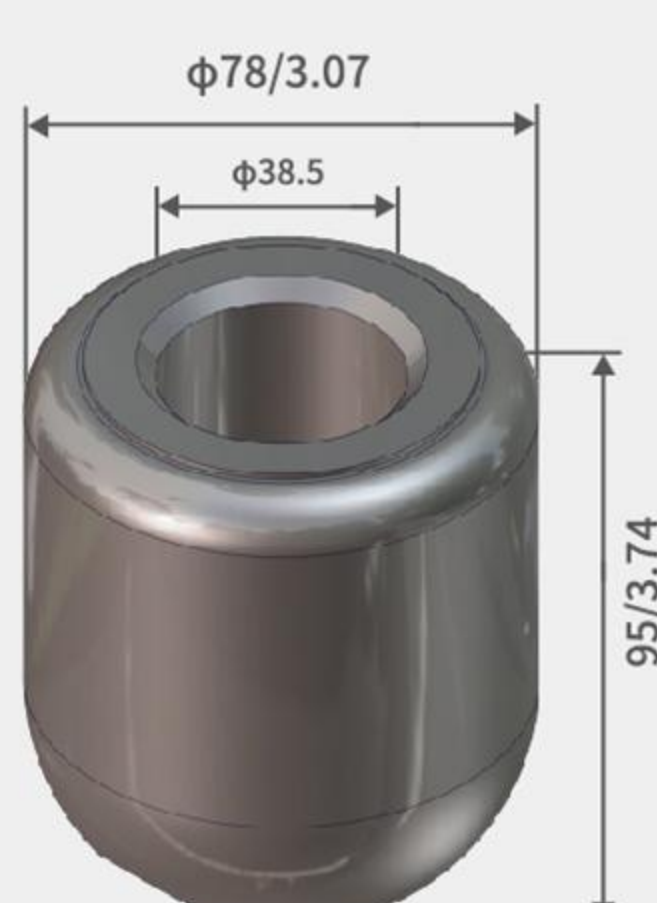
大圆座78-95
