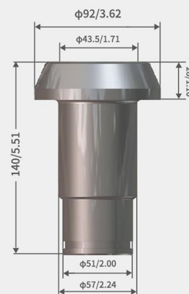
U170齿套
